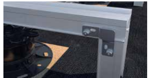
Anwendungsbeispiel 90° Profilverbinder
