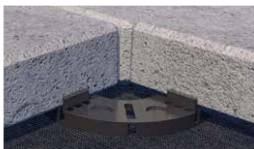
Anwendungsbeispiel Plattenlager PP
