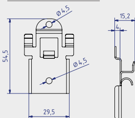
Fassadenclip-Rhombus
