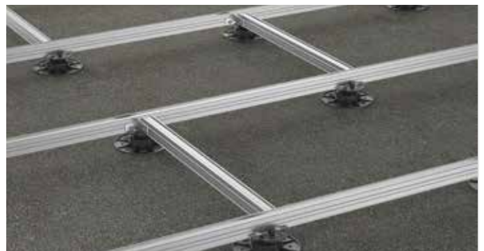
Verstellfuß BASE mit Alu-Systemprofil EVO Light
